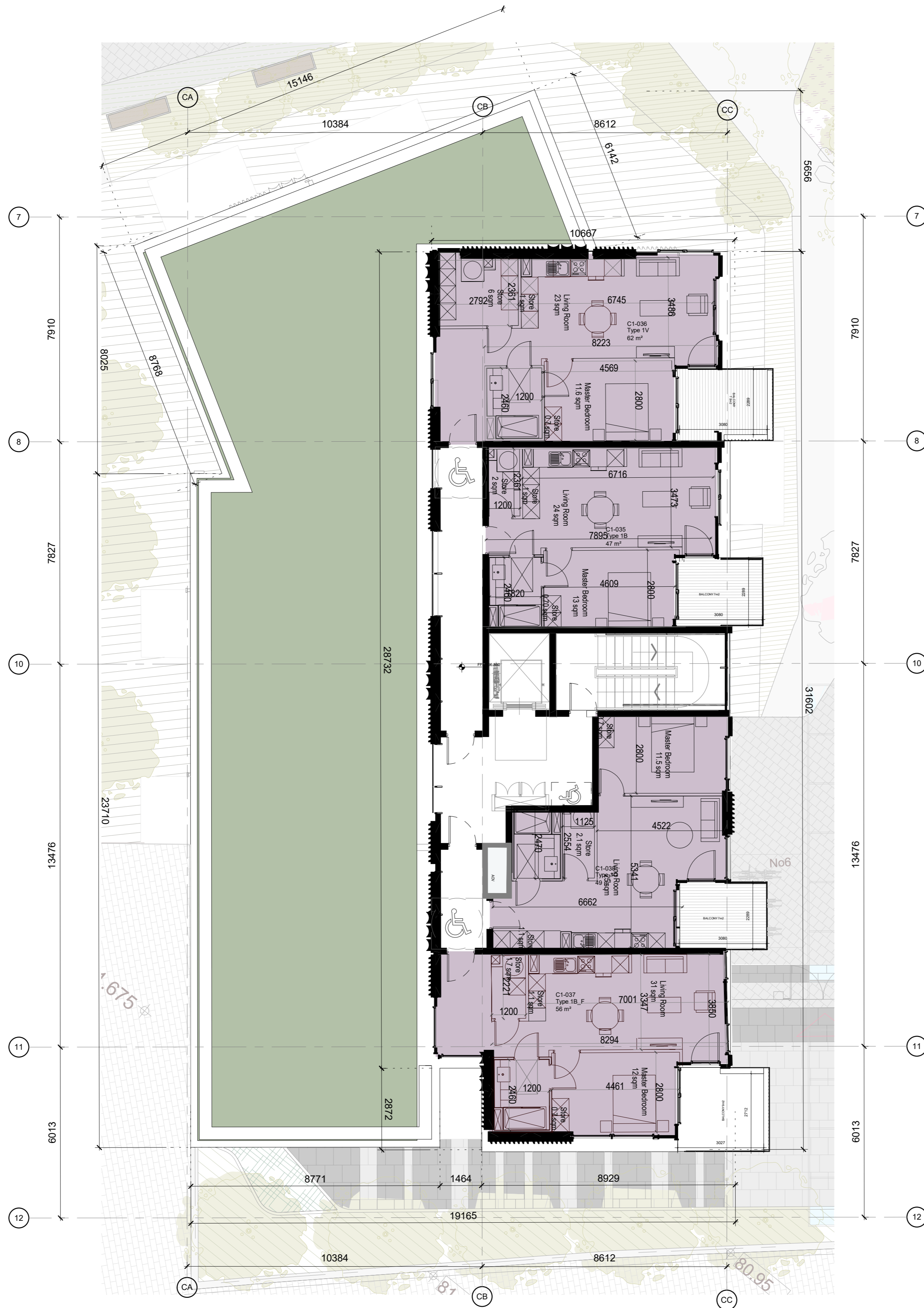
1 05 FFL GA Part V Block C 1 : 100
